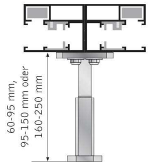
Abstandhalter für ein oder zwei Führungsschienen
