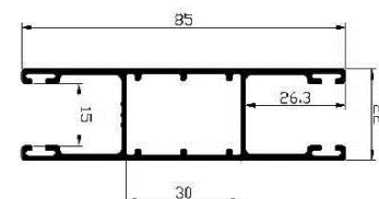
DF3 (Doppel-Führungsschiene)
