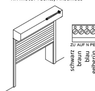
RR Motor rechts, Anschluss
