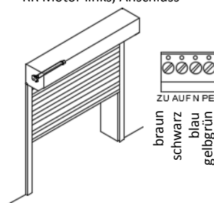
RR Motor links, Anschluss
