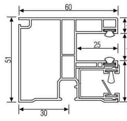
PVC-FS für ISG (einfach)
