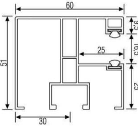
ALU-FS f. Maxi-Profil, einfach
