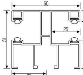
ALU-FS f. Maxi-Profil, doppelt
