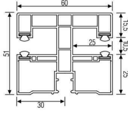
PVC-FS f. Maxi-Profil, doppelt
