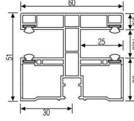
PVC-FS f. Maxi-Profil, doppelt
