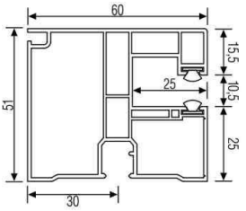
PVC-FS f. Maxi-Profil, einfach
