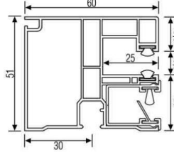
PVC-FS für ISG (einfach)
