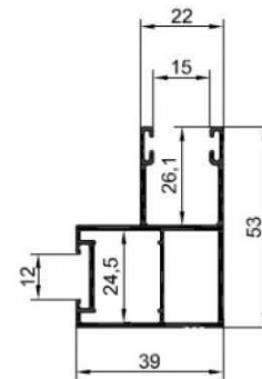
Distanz-FS 53mm (Aufpreis) zur Kombination mit ISG-Element
