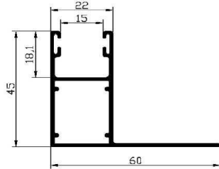
A6 – RR-FS, schmal (o. Aufpreis)
