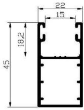
A5-FS, schmal 45mm (o. Aufpreis)
