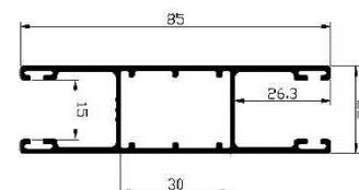
DF3 (Doppel-Führungsschiene)
