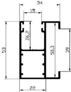
A3-12mm Abstands-FS 53mm (Aufpreis)
