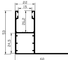
A3 (Standard-Führungsschiene) A4 (Rechtsroller-Führungsschiene)
