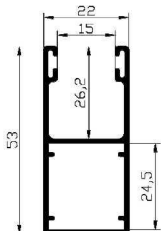
A3 (Standard-Führungsschiene) A4 (Rechtsroller-Führungsschiene)
